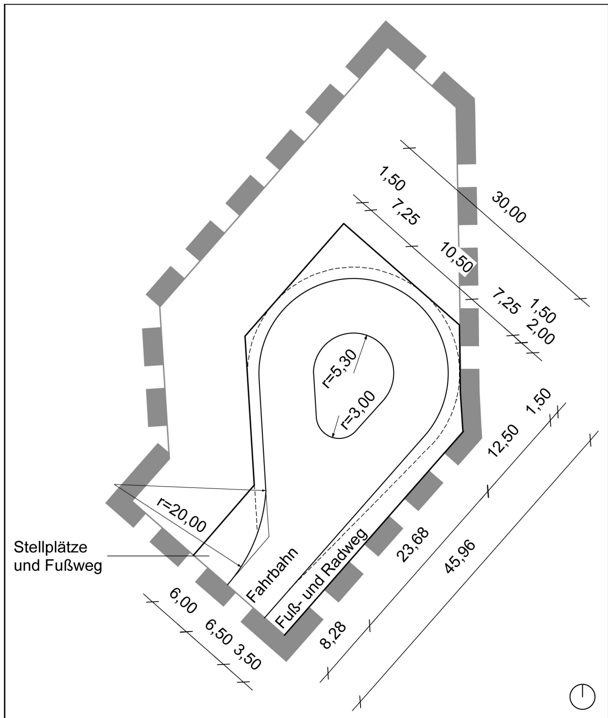
Abbildung 1: Zeichnung von studio nelke zur möglichen Lage eines Wendekreises für Lastzüge gemäß RAST06 innerhalb der geplanten Straßenverkehrsflächen
