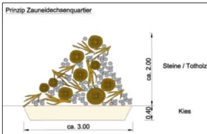
Abbildung 3: Prinzipskizze Zauneidechsenquartiere
